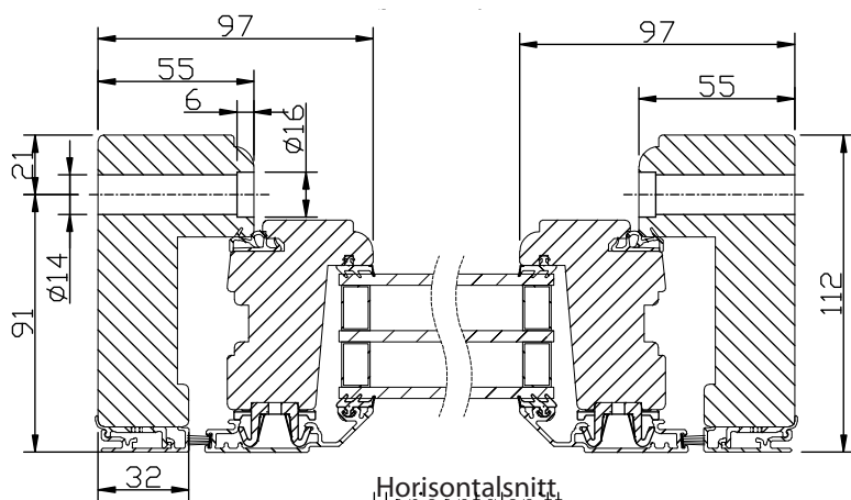
Horizontalsnitt bågpost
