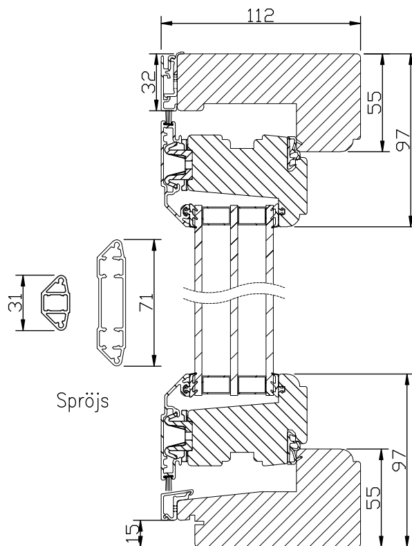
Vertikalsnitt Vertikalsnitt
