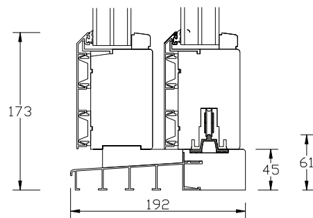
Vertikalsnitt Typ C Aluminium
