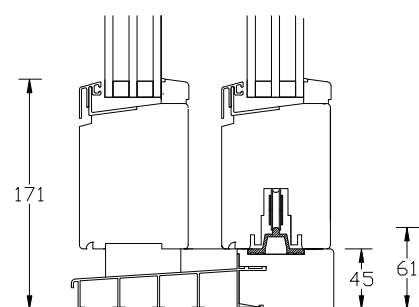
Vertikalsnitt Typ A Trä
