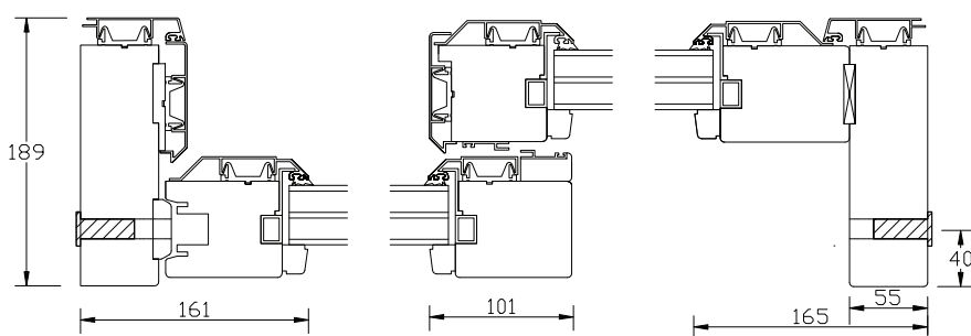
Horizontalsnitt Typ A Aluminium
