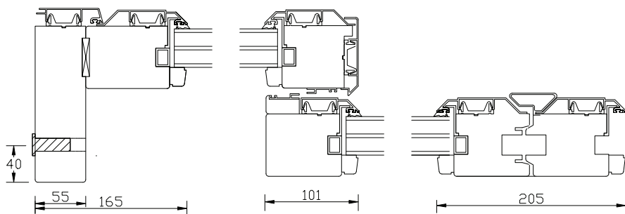
Horizontalsnitt Typ C Aluminium
