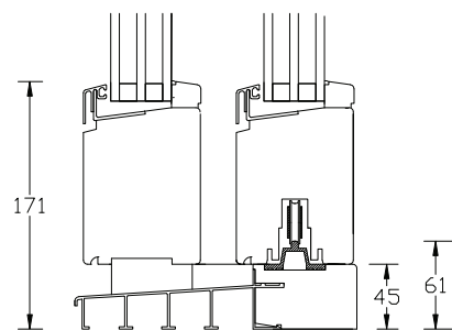
Vertikalsnitt Typ C Trä
