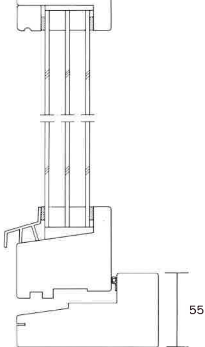
Snitt A2-A2
