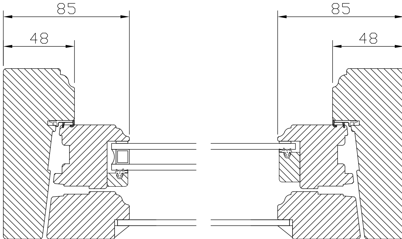
Horizontalschnitt
