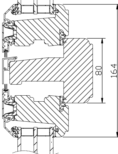
Vertikalsnitt karm tvärpost
