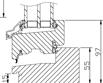
Vertikalsnitt
