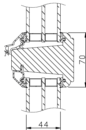
Vertikalsnitt bågpost
