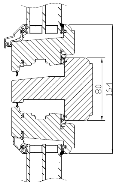
Vertikalsnitt Tvärpost
