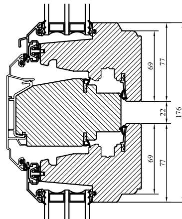
Vertikalsnitt karm tvärpost
