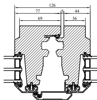
Horizontalsnitt mötesbåge
