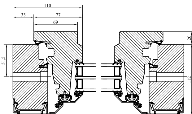
Horizontalsnitt
