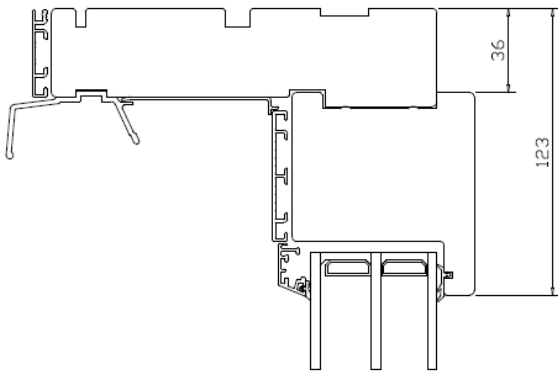
Vertikalsnitt Aluminium
