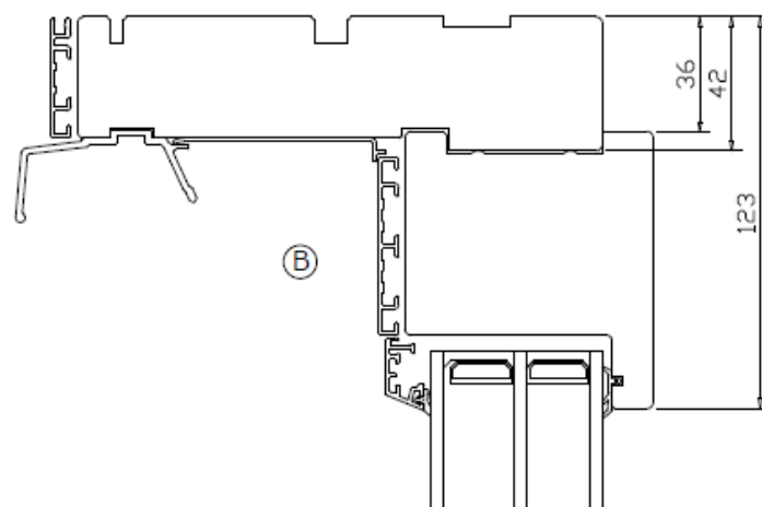
Vertikalsnitt B - I - D (fast del)
