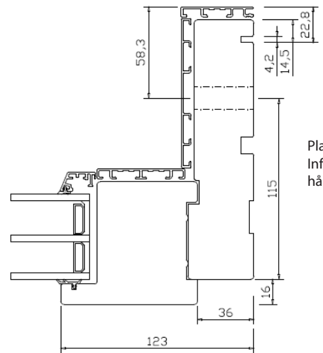
Horizontalsnitt Aluminium
