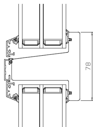
Bågpost I - I
