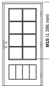
Glashöjd 15 Spröjs 3:1
