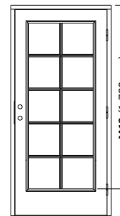
Glashöjd 19 Spröjs 4:1
