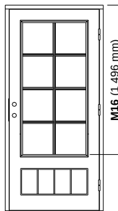
Glashöjd 16 Spröjs 3:1
