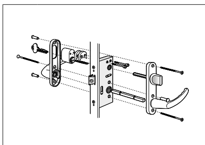
Alt 3: Fönsterdörr Spärrvred insida, cylinder utsida
