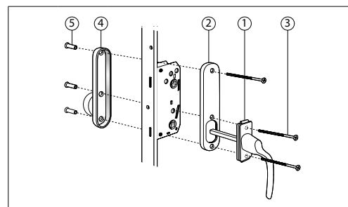
Alt 5: Fönsterdörr standard. Barnspärr insida, Draghandtag utsida
