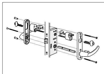
Alt 4: Fönsterdörr Cylinder insida, cylinder utsida
