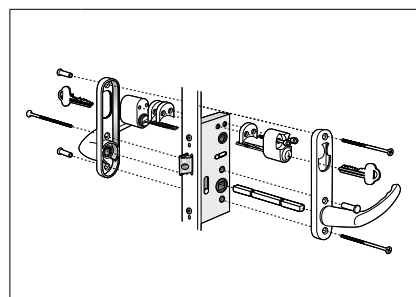
Alt 4: Fönsterdörr Cylinder insida, cylinder utsida
