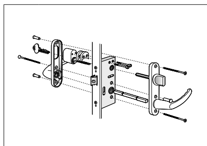
Alt 3: Fönsterdörr Spärrvred insida, cylinder utsida
