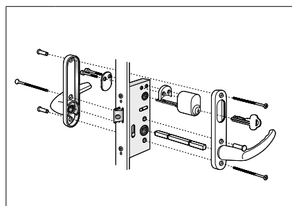
Alt 2: Fönsterdörr Cylinder insida, täckbricka utsida
