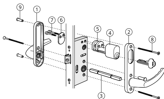
Alt 2: Fönsterdörr Cylinder insida, täckbricka utsida.
