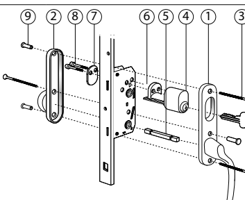
Alt 5:5: Fönsterdörr Cylinder insida, Draghandtag utsida
