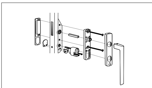
Skjutdörr, alu. Cylinder insida, täckbricka utsida
