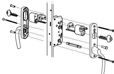
Alt 5:4: Fönsterdörr Cylinder insida, cylinder utsida.
