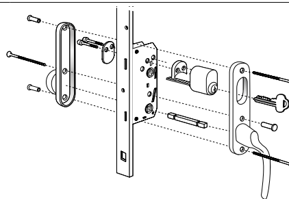
Alt 5:5: Fönsterdörr Cylinder insida, draghandtag utsida.
