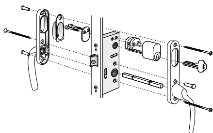
Alt 5:2: Fönsterdörr Cylinder insida, handtag utsida.
