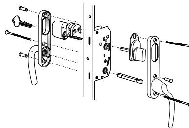
Alt 5:3: Fönsterdörr Spärrvred insida, cylinder utsida.
