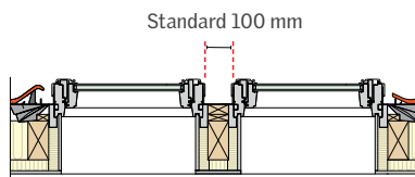
Bilden visar ett standard 100 mm montage där befintlig takstol behålls.
