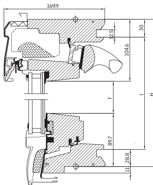
Vertikal sektion
