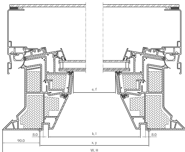
Horisontell sektion
